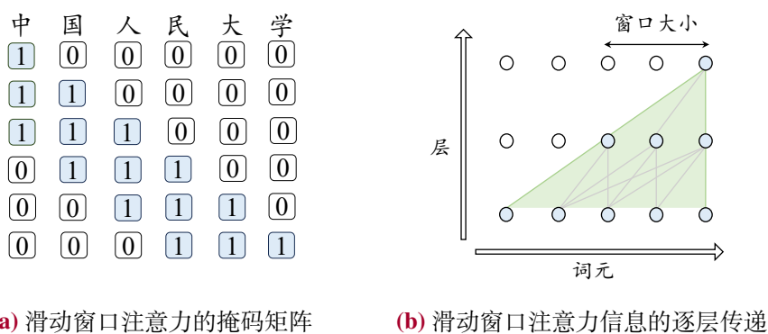
图 5.3 滑动窗口注意力示意图
